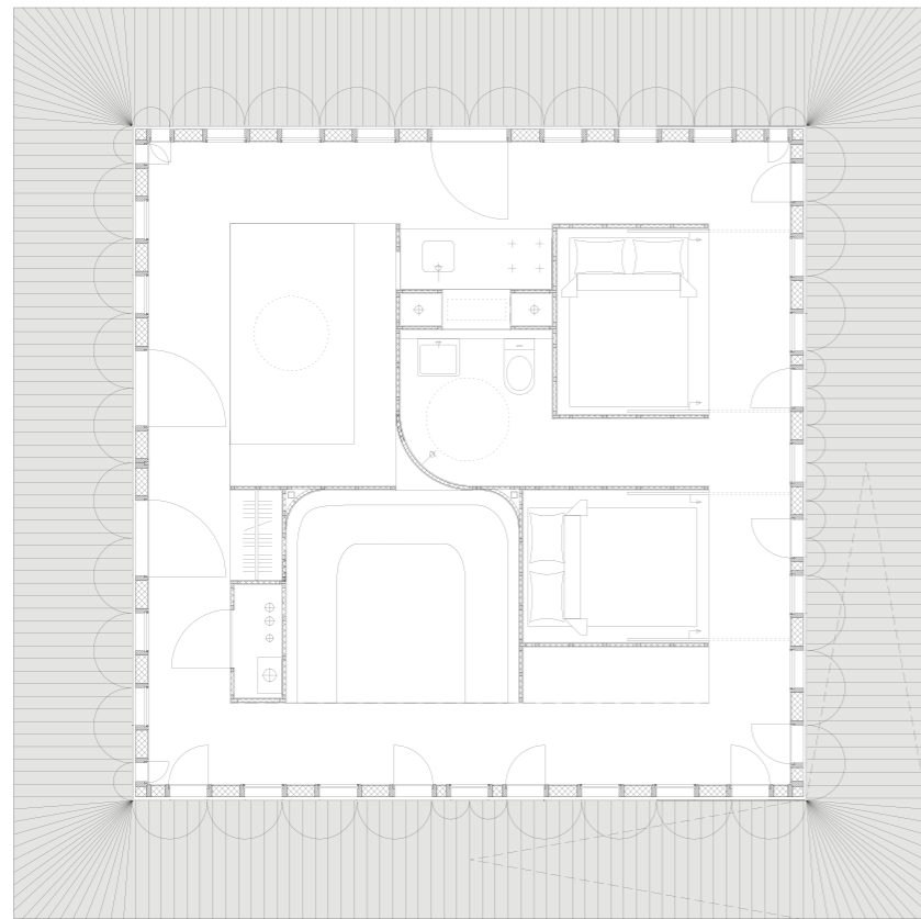
MGR-plattegrond 1:50
